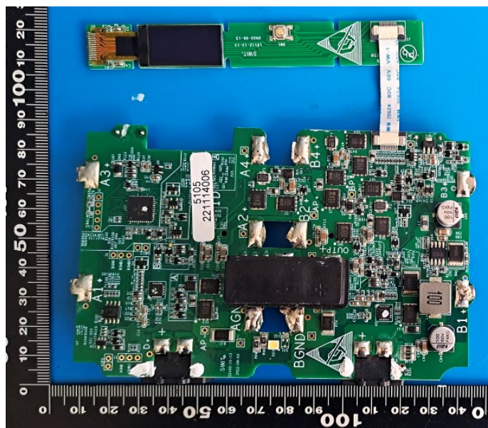
Fig. 6 – Back view of PCM 表6 – PCM 反面视图
